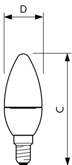
B40 220-240V 8.5-60W 806lm 27-22K E14
